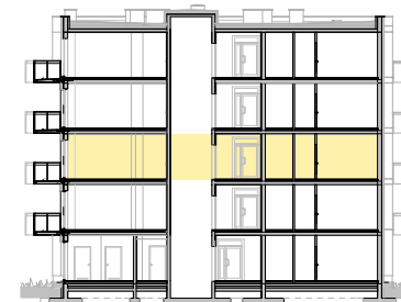
przekrój
